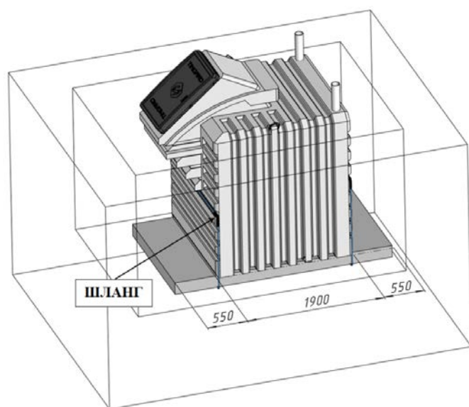
Рисунок 4 – Установка погреба
